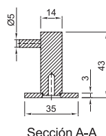
Sección A-A
