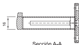
Sección A-A
