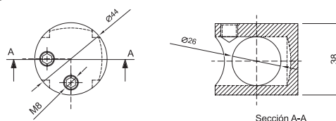
Nudo T 90°+90°
